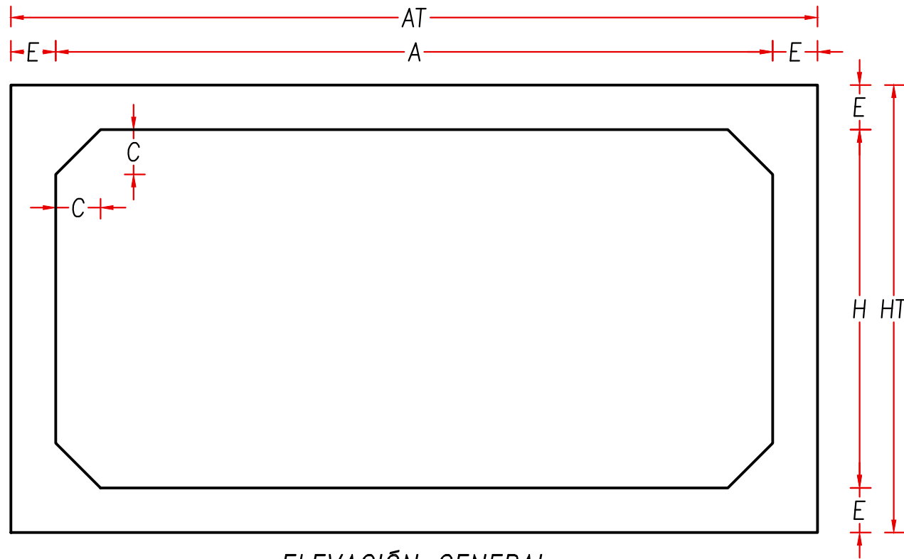
ELEVACIÓN GENERAL ESC. 1/30
