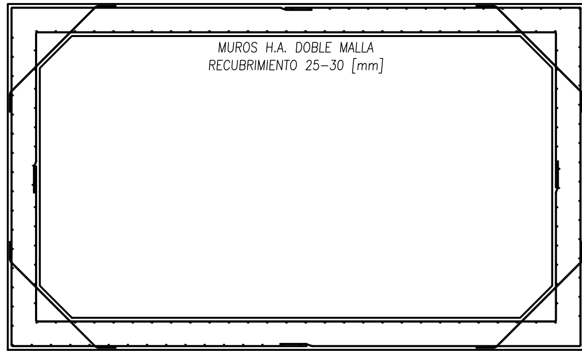
ARMADURA ELEVACIÓN GENERAL ESC. 1/30
