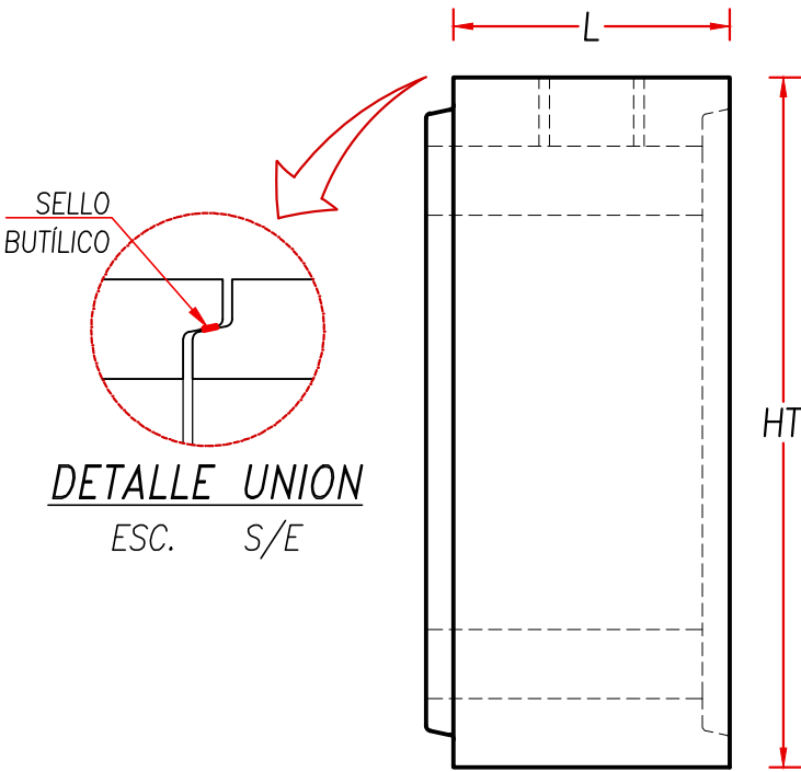
ELEVACIÓN VISTA LATERAL ESC. 1/30
