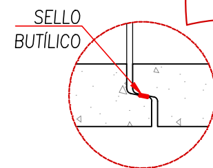
DETALLE UNION ESC. S/E
