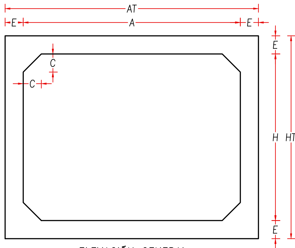
ELEVACIÓN GENERAL ESC. 1/30
