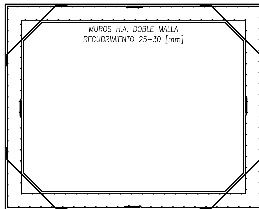
ARMADURA ELEVACIÓN GENERAL ESC. 1/30
