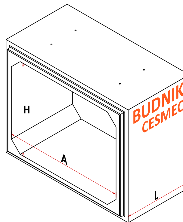
VISTA ISOMETRICA ESC. S/E
