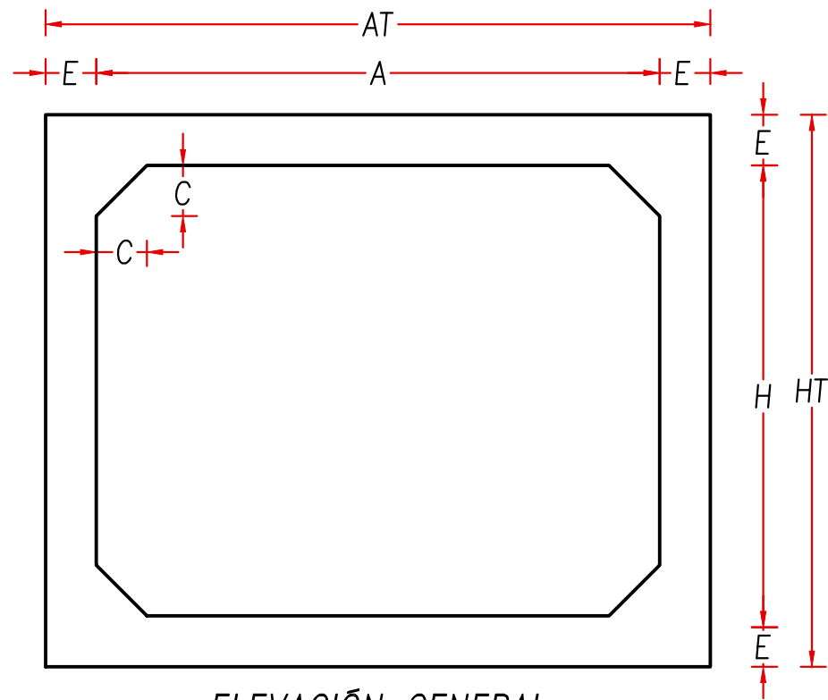
ELEVACIÓN GENERAL ESC. 1/30
