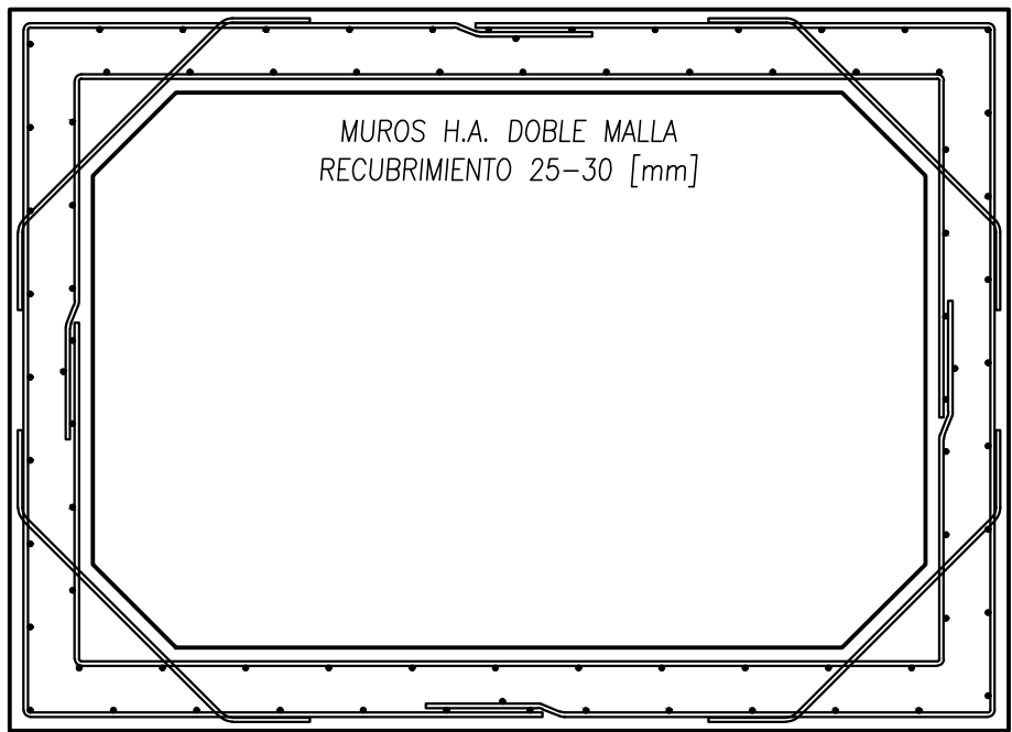
ARMADURA ELEVACIÓN GENERAL ESC. 1/15
