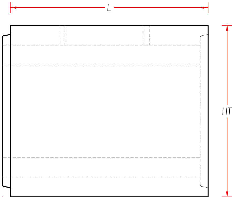
ELEVACIÓN VISTA LATERAL ESC. 1/15
