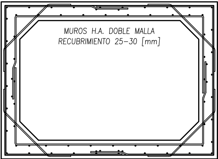
ARMADURA ELEVACIÓN GENERAL ESC. 1/15
