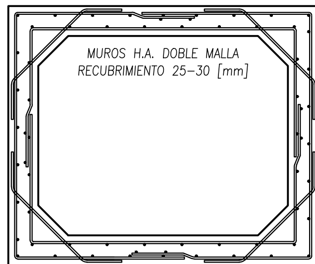
ARMADURA ELEVACIÓN GENERAL ESC. 1/15
