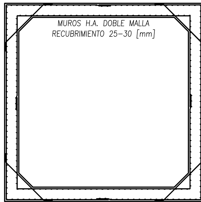
ARMADURA ELEVACIÓN GENERAL ESC. S/E
