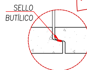
DETALLE UNION ESC. S/E
