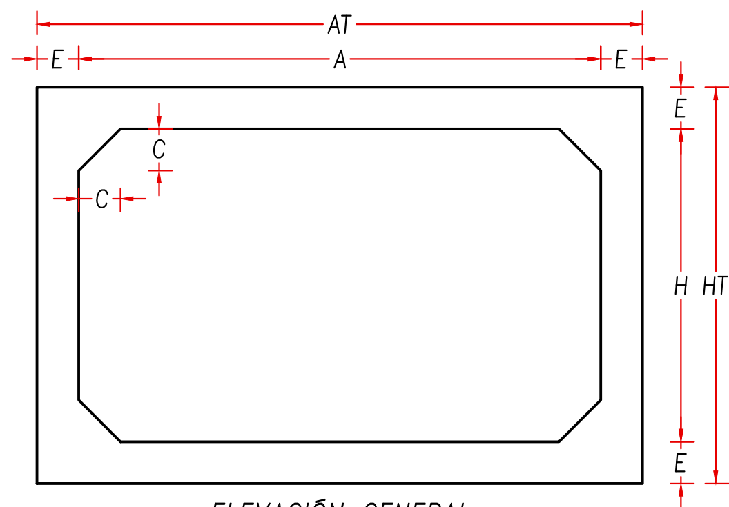
ELEVACIÓN GENERAL ESC. 1/25
