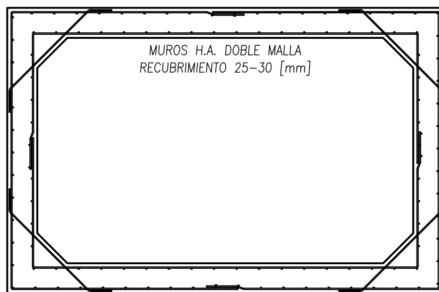
ARMADURA ELEVACIÓN GENERAL ESC. 1/25
