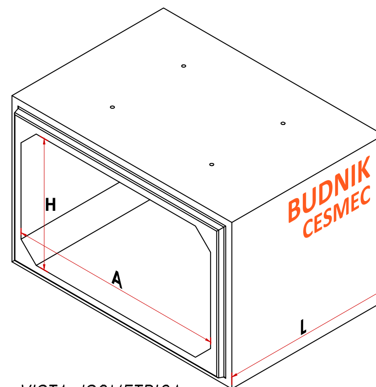
VISTA ISOMETRICA ESC. S/E
