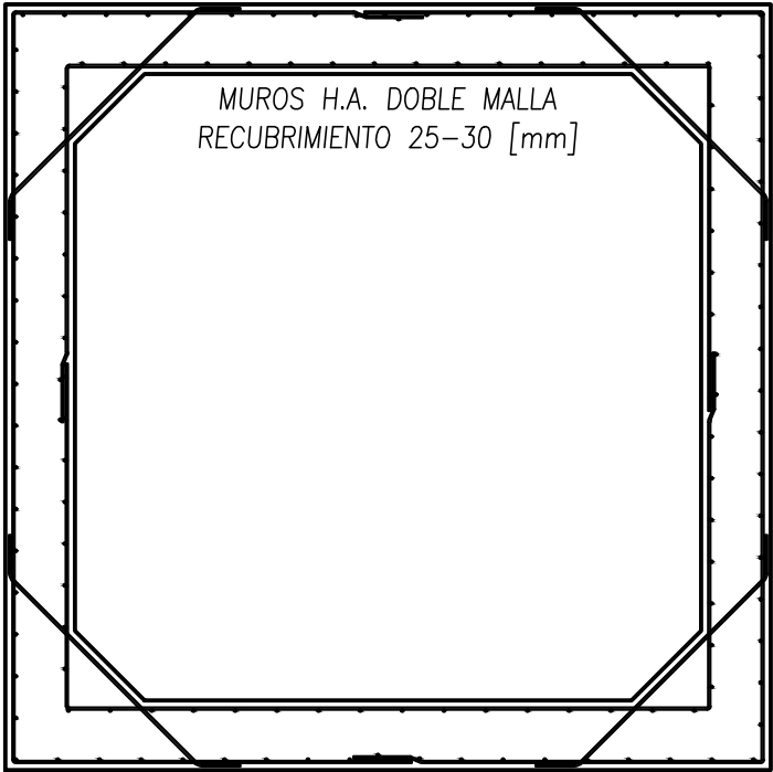
ARMADURA ELEVACIÓN GENERAL ESC. 1/30
