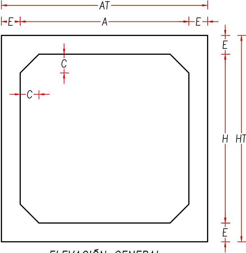
ELEVACIÓN GENERAL ESC. 1/30
