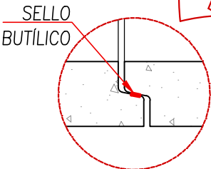
DETALLE UNION ESC. S/E
