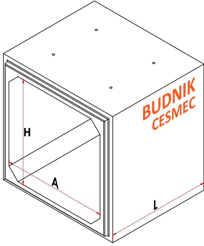
VISTA ISOMETRICA ESC. S/E
