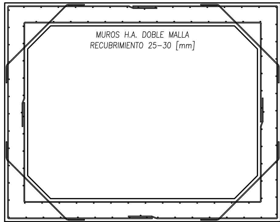
ARMADURA ELEVACIÓN GENERAL ESC. 1/20
