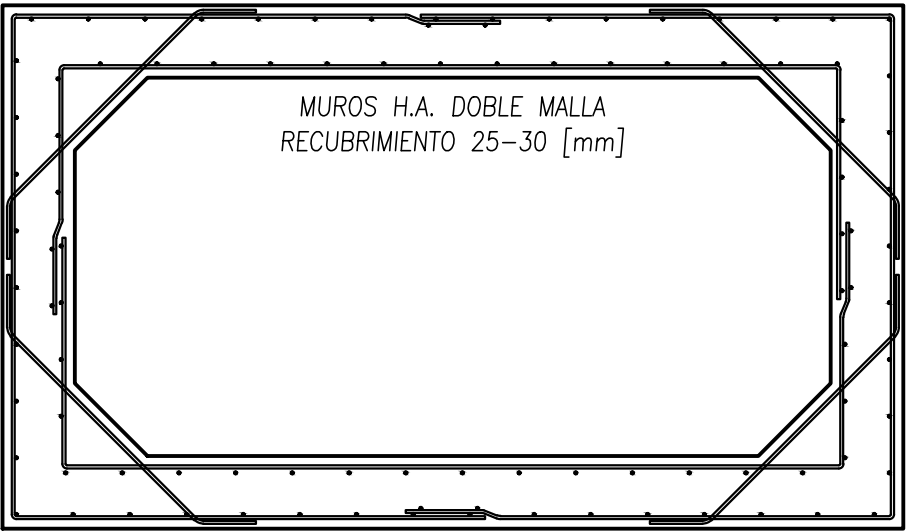
ARMADURA ELEVACIÓN GENERAL ESC. 1/20
