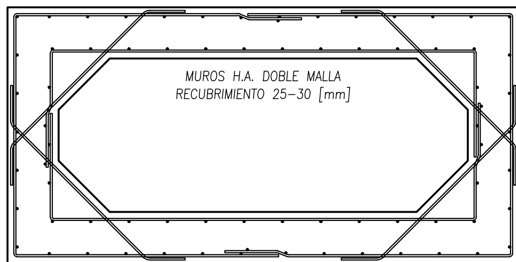
ARMADURA ELEVACIÓN GENERAL ESC. 1/15
