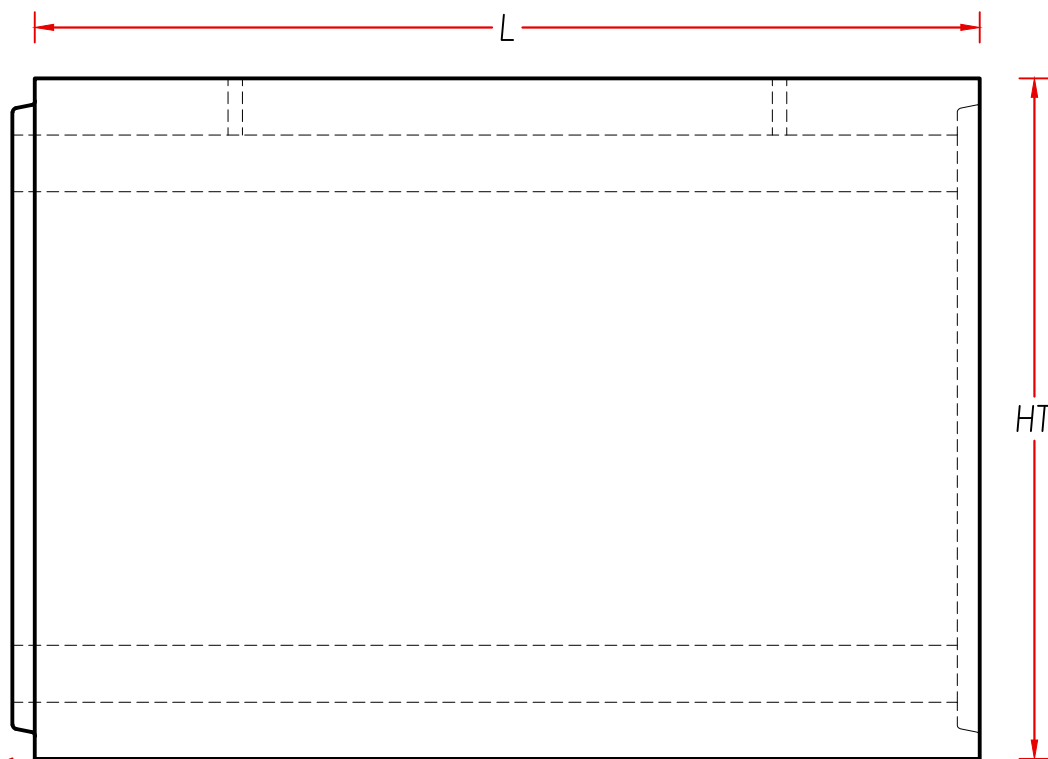
ELEVACIÓN VISTA LATERAL ESC. 1/20
