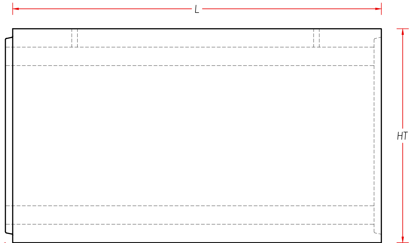
ELEVACIÓN VISTA LATERAL ESC. 1/15
