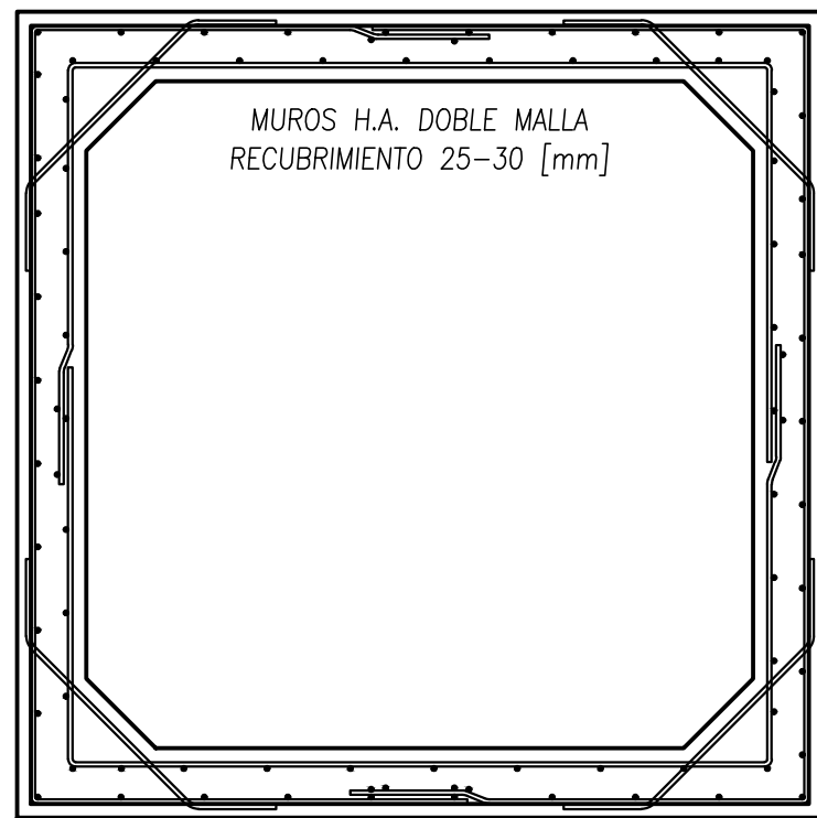
ARMADURA ELEVACIÓN GENERAL ESC. 1/15
