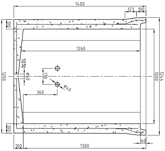
ELEVACION CAMARA
