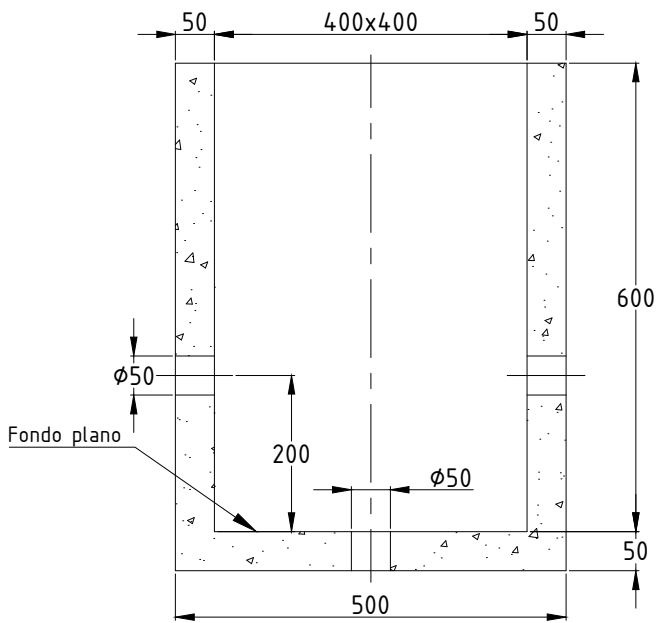
ELEVACION EN CORTE
