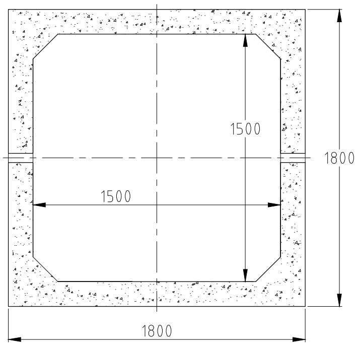
SECCION PLANTA \text{\textcircled{A}}
