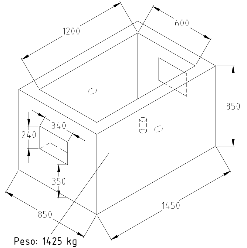
ISOMETRICA
