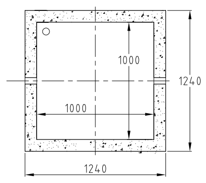
SECCION PLANTA
