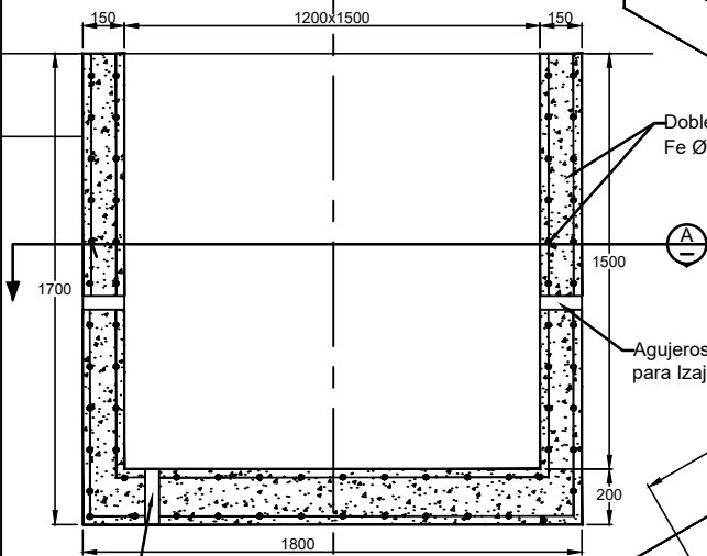
ELEVACIÓN
